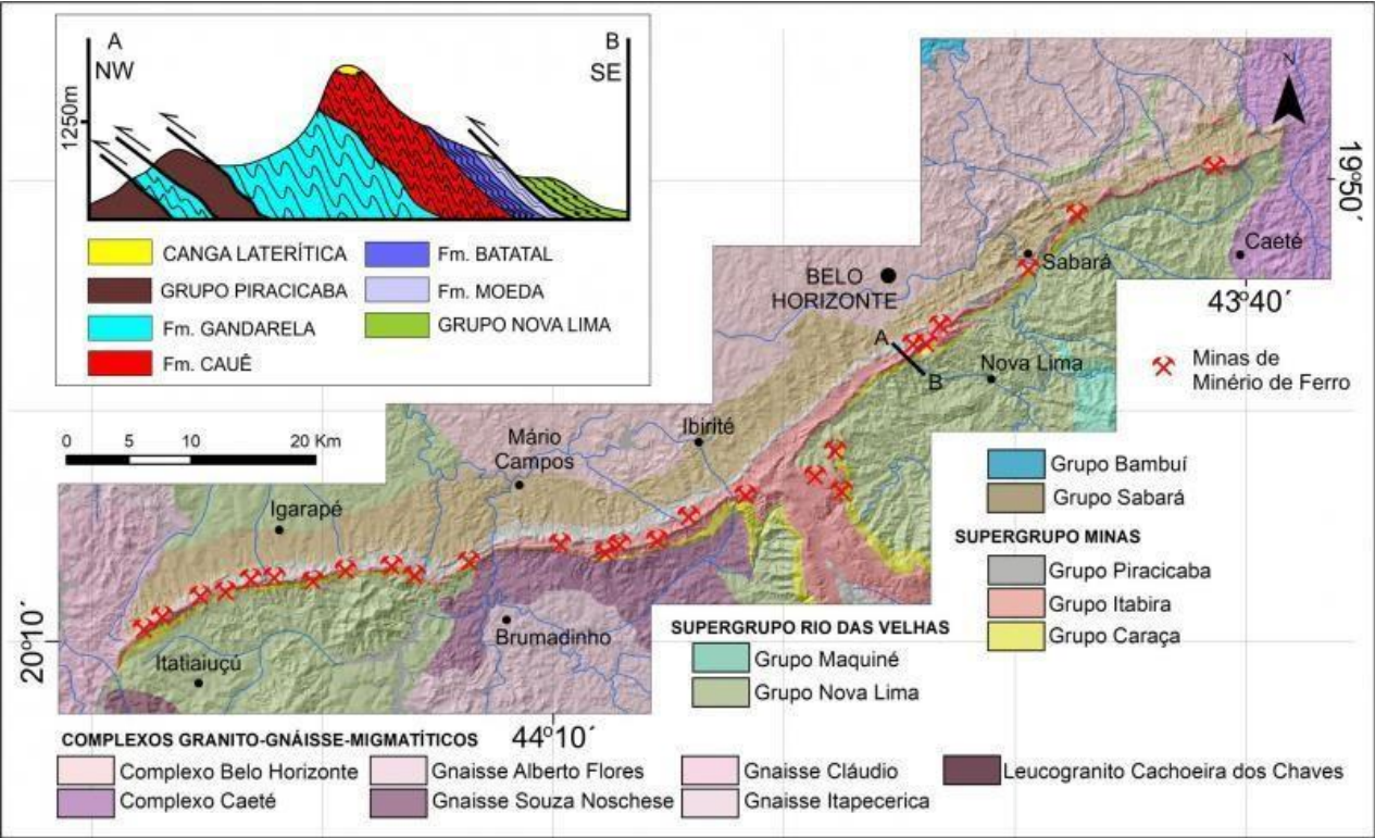
Figura 3 - Mapa geológico simplificado as Serra do Curral com a localização das minas de minério de ferro e perfil geológico de detalhe próximo a Mina de Águas Claras. Fonte: Cavalcanti, 2021.
